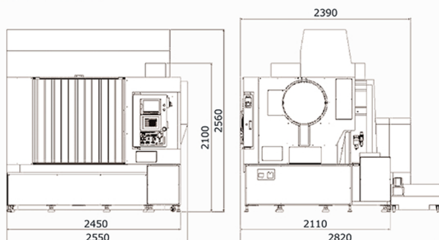
外形寸法図
